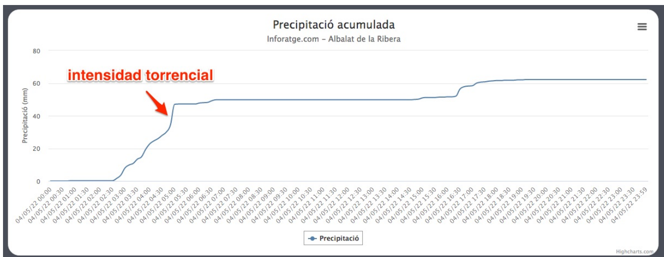
Evolución lluvia acumulada en ALBALAT DE LA RIBERA el día 04/05/22 (en l/m 2 ) https://inforatge.com/meteo-albalatdelaribera
