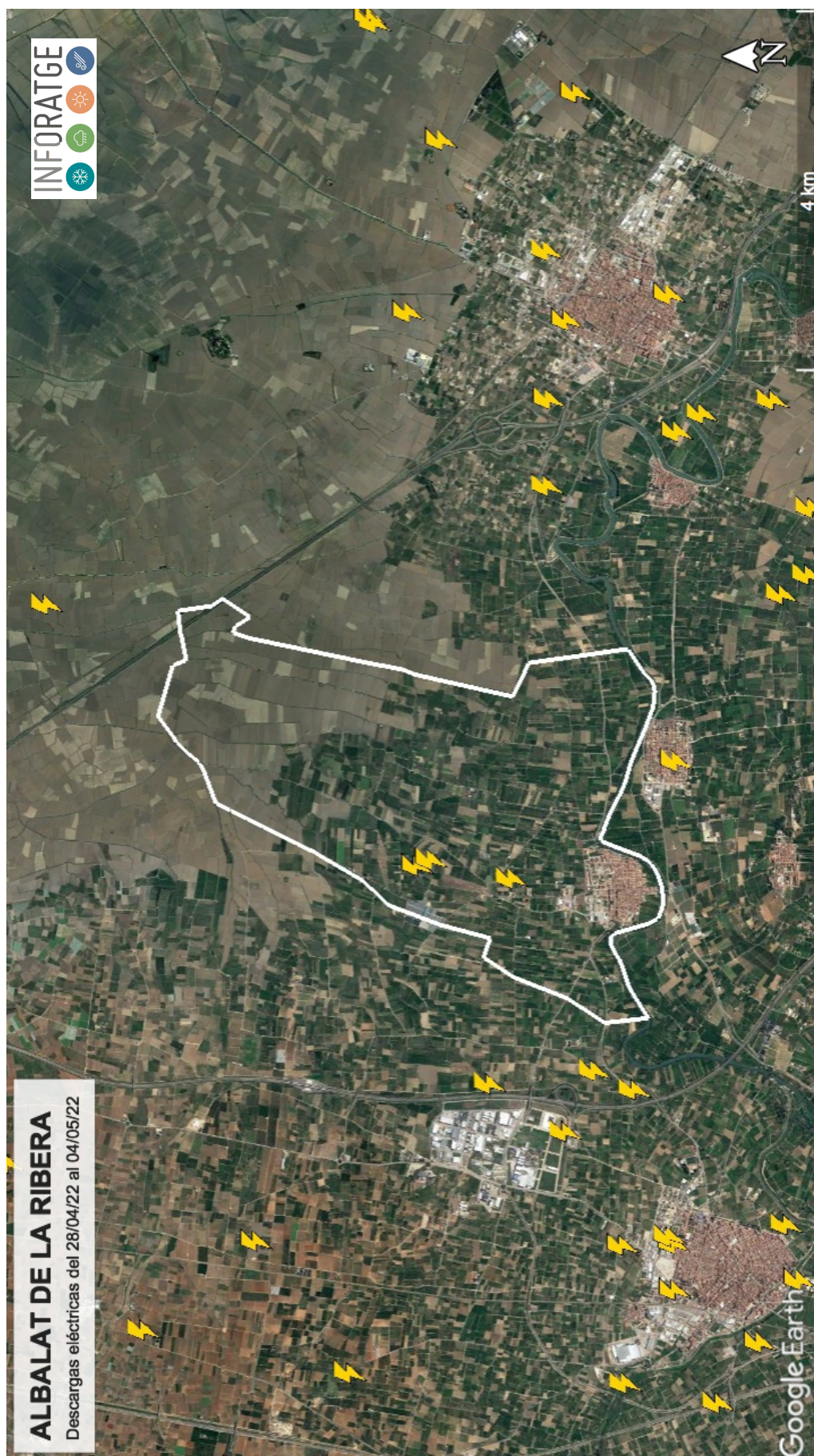
Descargas eléctricas ` nube-tierra` registradas en el término municipal de ALBALAT DE LA RIBERA y alrededores entre el 28/04/22 y el 04/05/22 Geolocalización descargas eléctricas: AEMET-Agencia Estatal de Meteorología // Cartografía: Instituto Geográfico Nacional de España
